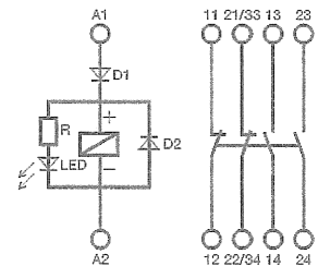
DTRS-468-1023/1024 内部接続図
