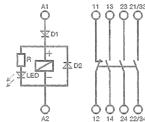
DTRS-468-1009/1010 内部接続図
